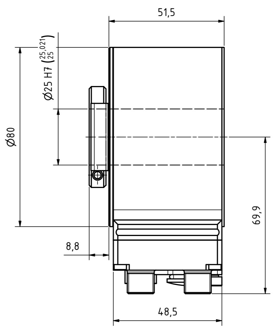
Ansicht A
