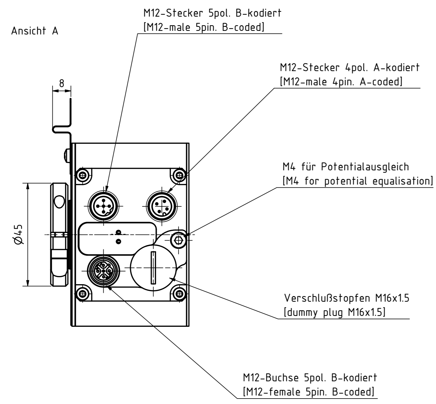
Ansicht A
