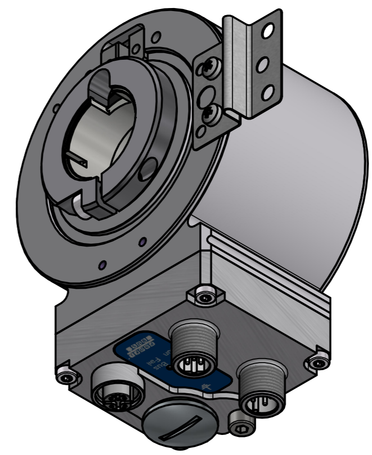
Isometrie ( 1 : 1 )
